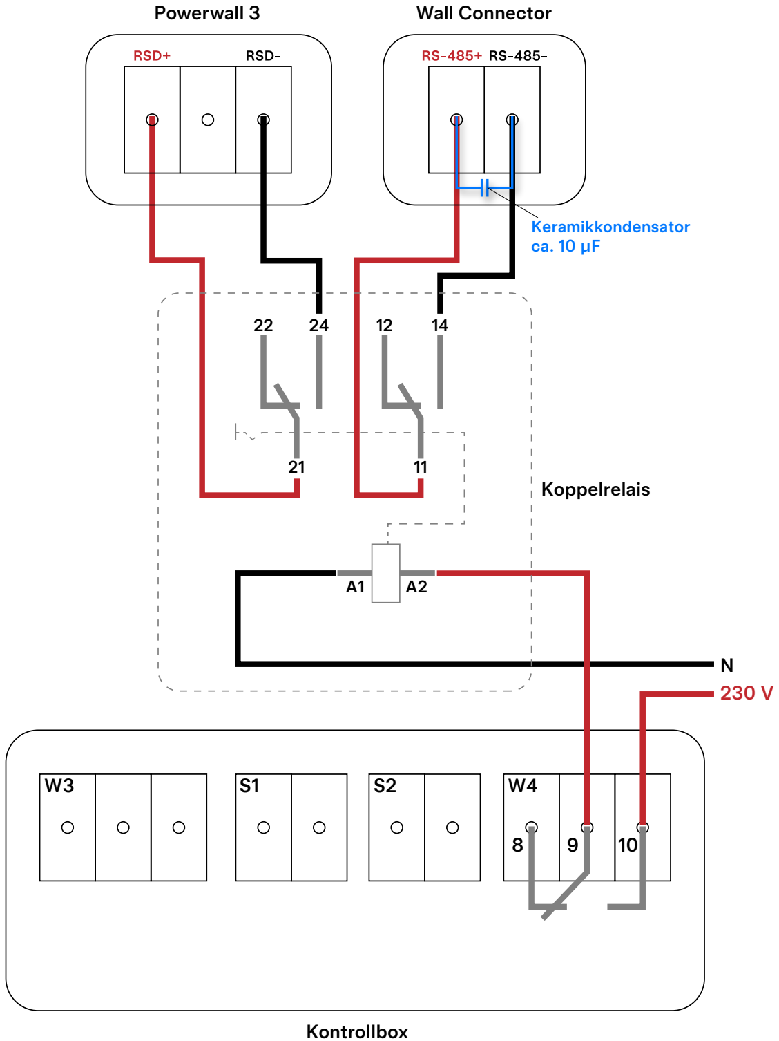
Abbildung 1. Einphasiger Übersichtsschauplan zum Anschluss von Wall Connector und Powerwall 3 an eine Kontrollbox via Koppelrelais.
